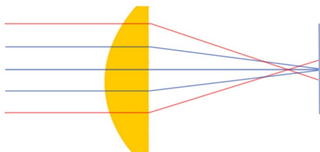
Sférické čočky
